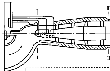
图 2 轴流式通风机测压断面位置图
