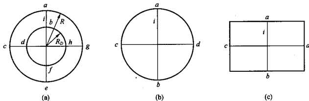
图 1 静压测点安装位置示意图
