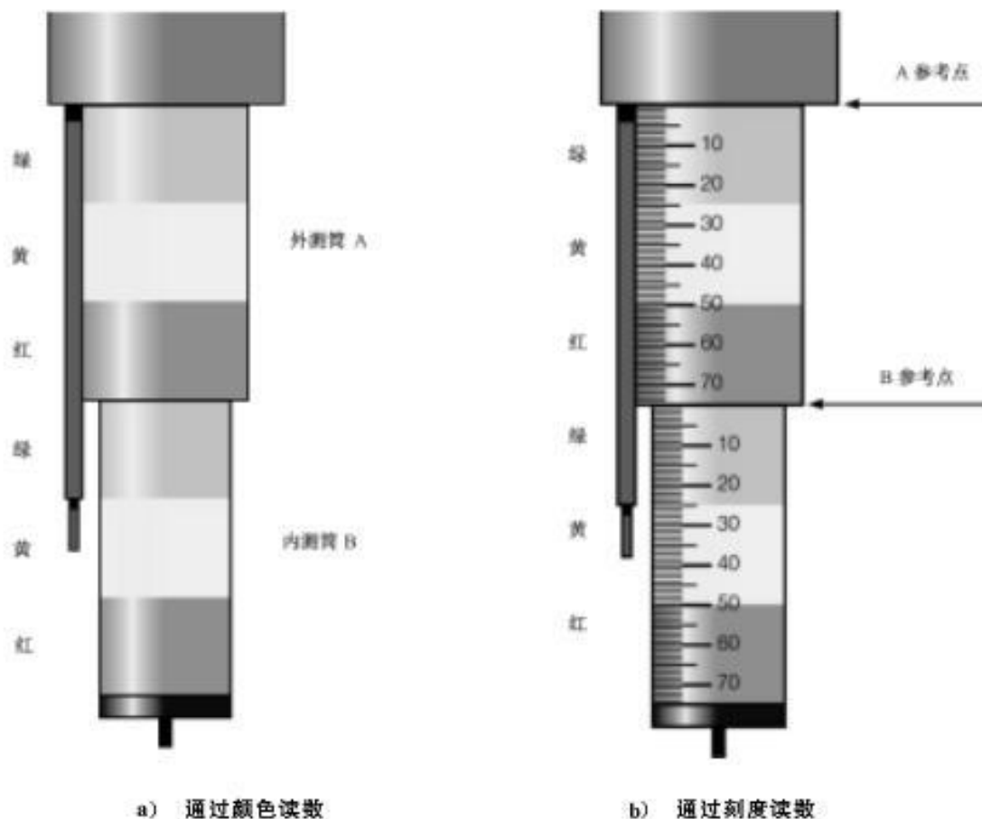
图 C.2 读数方法
